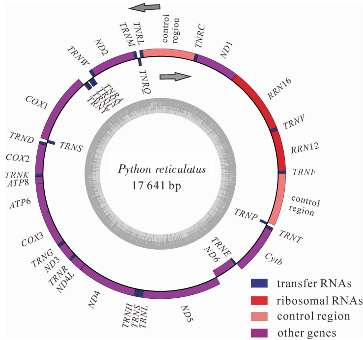
图 1 网纹蟒线粒体基因组结构示意图
