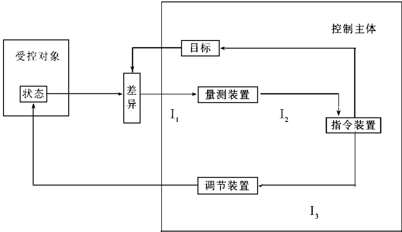
图 3 一般的反馈控制系统
