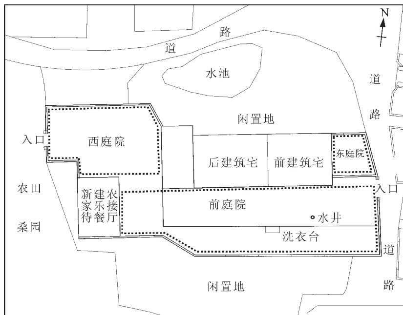
图1 改造前农家庭院平面图
