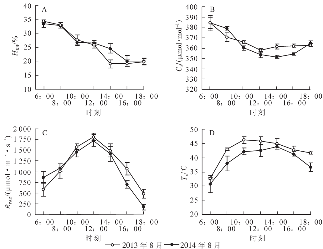
图 1 2014 年 8 月、2013 年 8 月环境因子日变化
