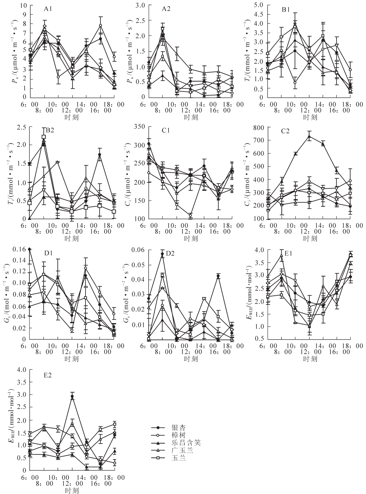
图4 高温条件下5个树种叶片净光合速率( P_n )蒸腾速率( T_r )胞间二氧化碳摩尔分数( C_i )气孔导度( G_s )和水分利用率( E_{\text{wue}} )日变化
