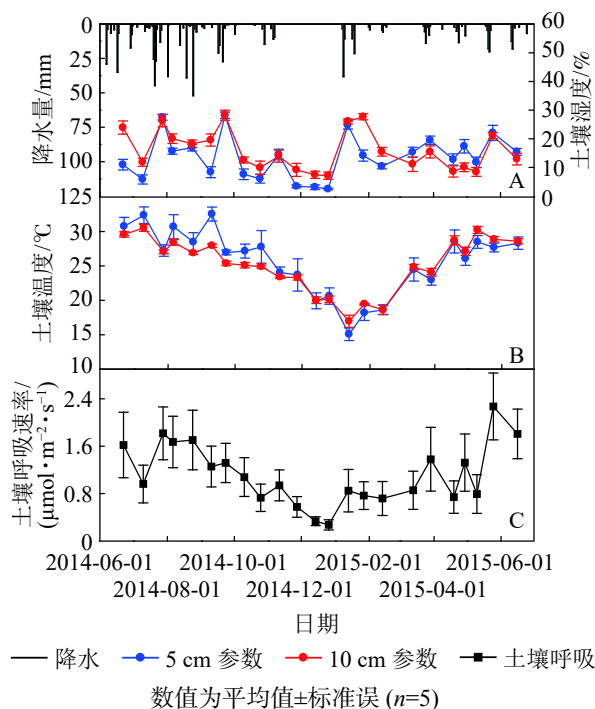
图1 2014年6月至2015年6月降水量, 土壤湿度(A), 土壤温度(B)和土壤呼吸速率(C)季节变化
