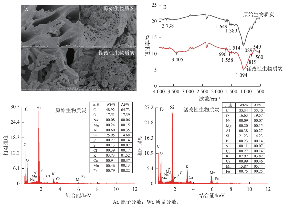
图1 改性前后生物质炭的扫描电镜图(A)、傅里叶红外光谱图(B)以及原始生物质炭X射线能谱分析图(C)和锰改性生物质炭X射线能谱分析图(D)
