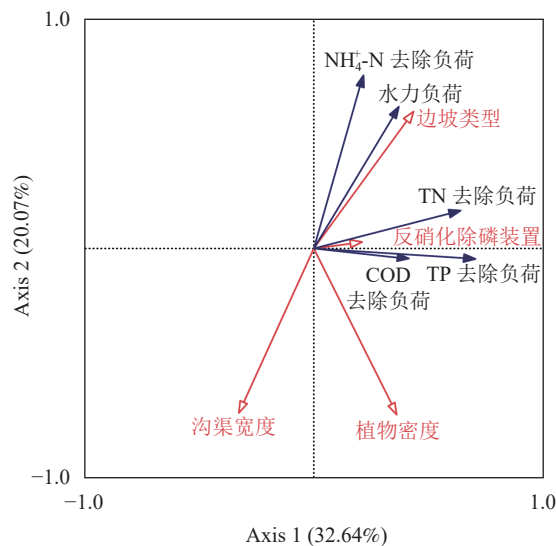
图4 不同生态沟渠类型对各农业面源污染物去除负荷的冗余分析
