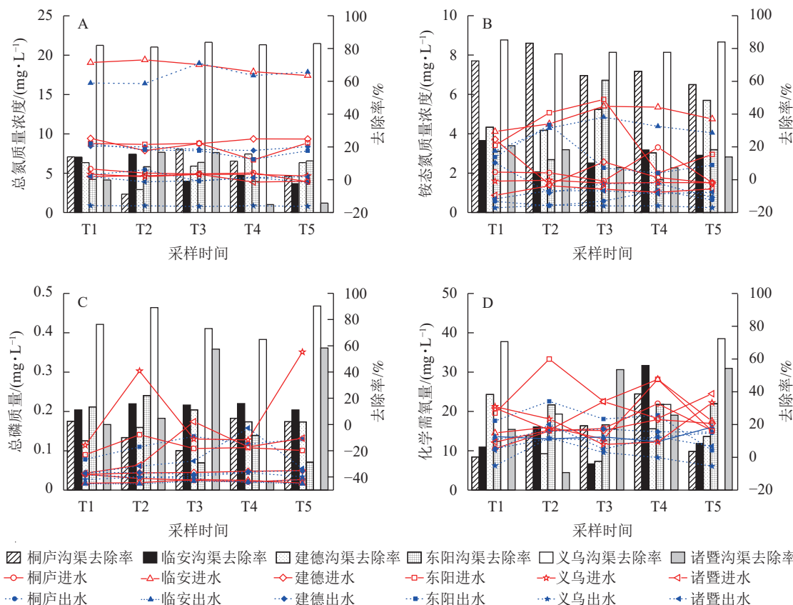
图 2 不同生态沟渠各农业面源污染物的进水质量浓度、出水质量浓度与去除率随时间的变化
