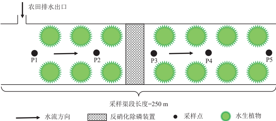
图 1 生态沟渠采样渠段取水点示意图
