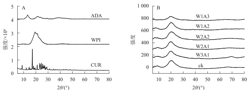
图 6 CUR、WPI、ADA(A) 和 WPI-ADA 微胶囊 (B) 的 XRD 谱图
