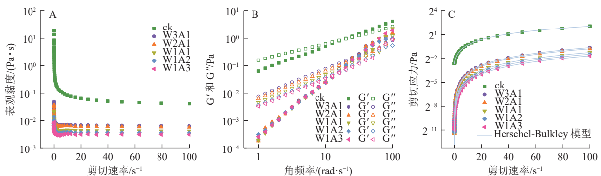
图 5 WPI-ADA 乳液表观黏度 (A)、频率扫描曲线 (B) 和剪切应力 (C)
