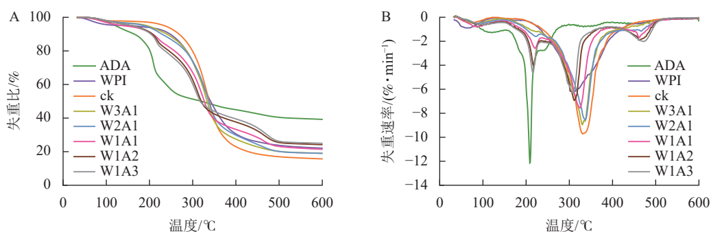
图 7 WPI-ADA 微胶囊的 TGA 曲线 (A) 和 DTG 曲线 (B)
