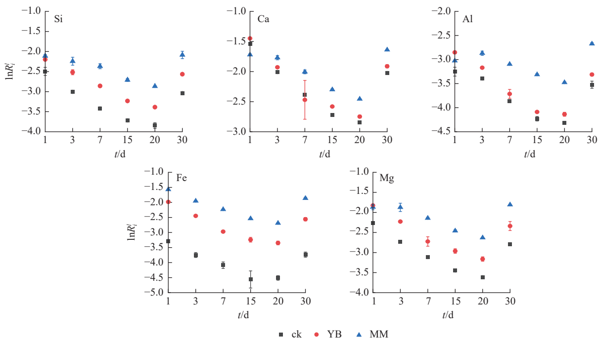
图5 浸提液中Si、Ca、Al、Fe、Mg的元素溶解速率随反应时间的变化
