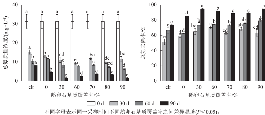
图 1 水中总氮质量浓度和对应去除率变化
