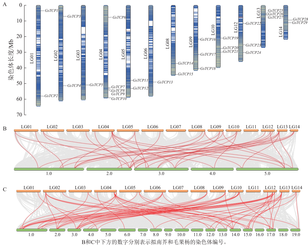
图 3 GsTCP 的染色体分布 (A)、皂荚与拟南芥 (B) 及毛果杨共线性 (C) 分析
