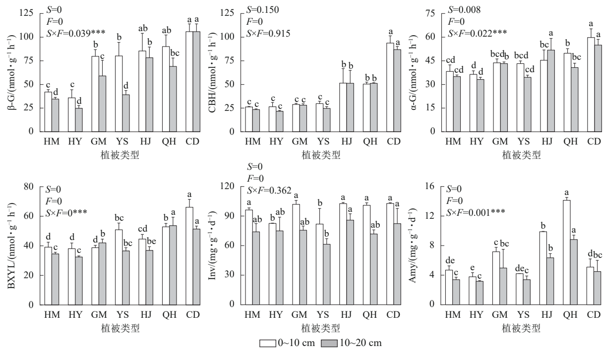
不同小写字母表示不同植被带土层间差异显著 ( P < 0.05 )；HM. 荒漠草原；HY. 灰榆；GM. 蒙古扁桃灌丛；YS. 油松；HJ. 云杉山杨混交林；QH. 青海云杉；CD. 亚高山草甸；S. 土壤；F. 植被； \beta -G. \beta -葡糖苷酶；CBH. 纤维二糖水解酶； \alpha -G. \alpha -葡糖苷酶活性；BXYL. \beta -木糖苷酶；Inv. 蔗糖酶；Amy. 淀粉酶。
