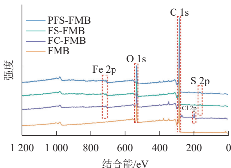
图 3 生物质炭的 X 射线光电子能谱分析 Figure 3 X-ray photoelectron spectroscopy analysis of biochars
