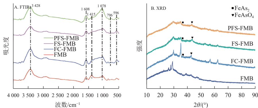
图 7 生物质炭吸附 As(III) 后的 FTIR 光谱和 XRD 衍射图谱
