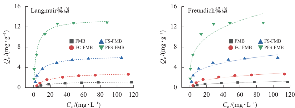
图 6 生物质炭对 As(III) 的等温吸附曲线
