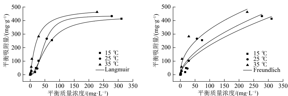
图 10 HPAAM-VIM-LS 对刚果红的吸附等温线模型
