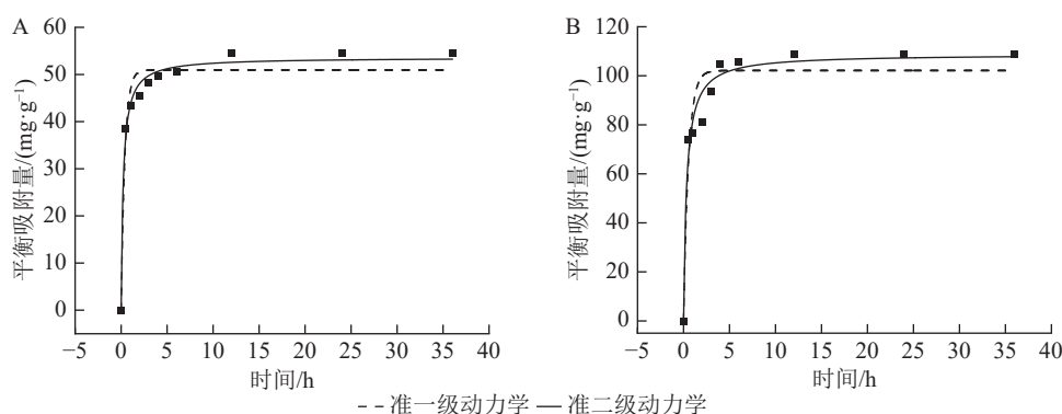
图 8 HPAAM-VIM-LS 对 100(A) 和 200\text{ mg}\cdot\text{L}^{-1} (B) 刚果红的吸附动力学拟合
