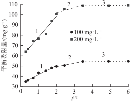
1、2、3 分别为吸附的阶段 1、阶段 2、阶段 3。
