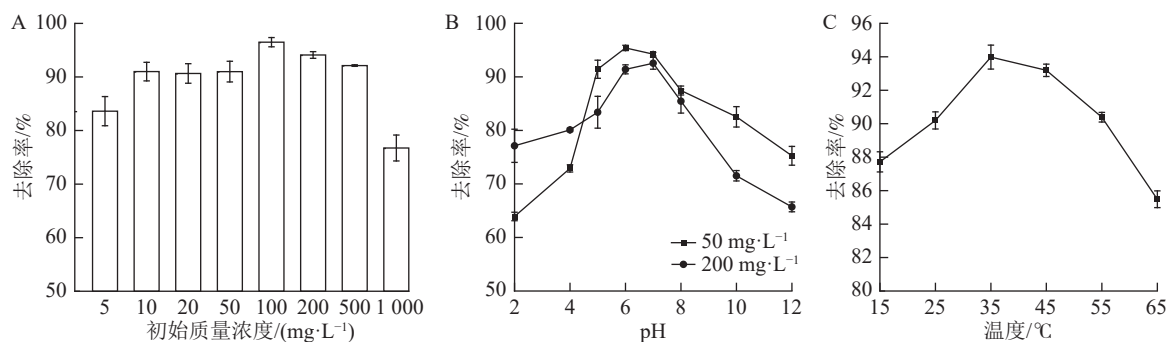
图 7 初始质量浓度、pH 和温度对 HPAAM-VIM-LS 吸附的影响
