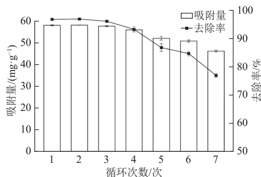
图 11 HPAAM-VIM-LS 对刚果红的重复吸附-解析循环
