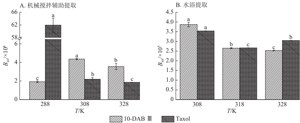
图 6 紫杉烷类化合物成分提取过程中 B_{10t} 与温度的关系
