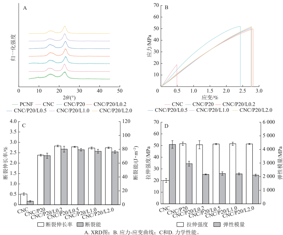
图3 CNC和CNC/PCNF/LNPs薄膜的XRD图、应力-应变曲线和力学性能
